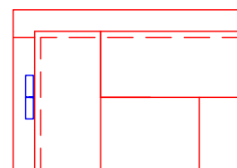
DETALLE SOLAPE HOJA-MARCO
